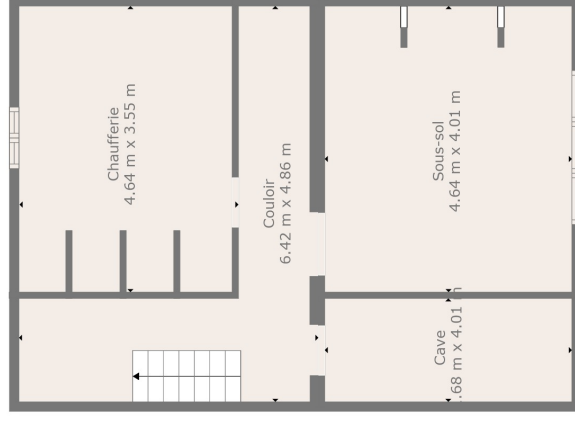
1er Étage
